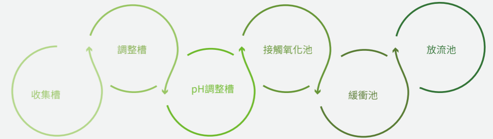
● 圖 2-12 六組製造後廢水處理水池槽圖
